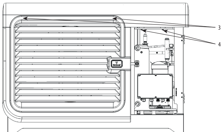
Rys. 57. Demontaż pokryw górną Airmax 3 - krok 2
