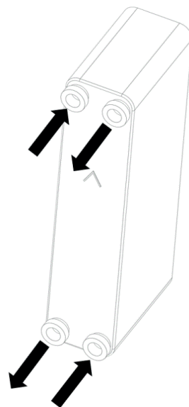
Rys. 73. Przeciwpądowe podłączenie wymiennika płytowego
