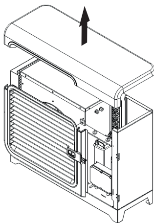
Rys. 58. Demontaż pokryw górną Airmax 3 - krok 3
