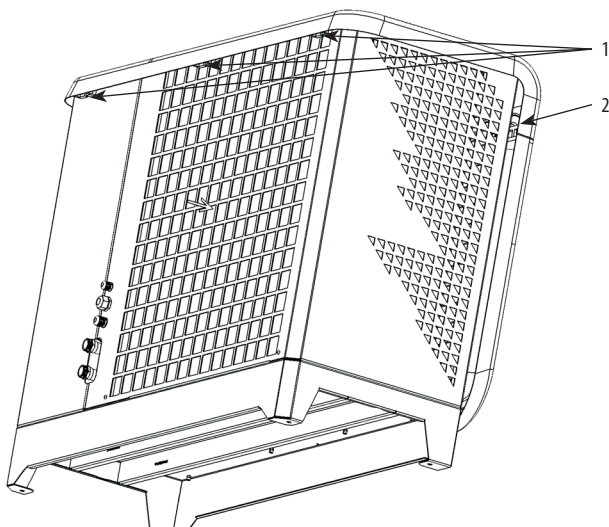
Rys. 56. Demontaż pokrywy górnej Airmax³ - krok 1
