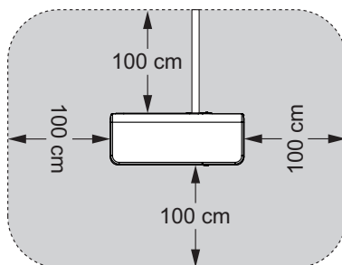
Rys. 35. Strefa ochronna pompy ciepła Airmax 3 - montaż wolnostojący
