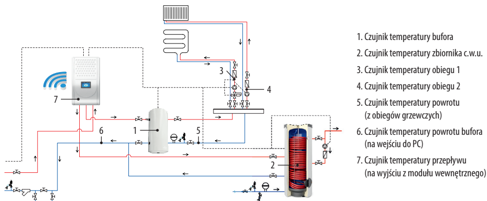
Rys. 106. Lokalizacja czujników związanych z obsługą obiegów hydraulicznych ogrzewania pomieszczeń i c.w.u.
