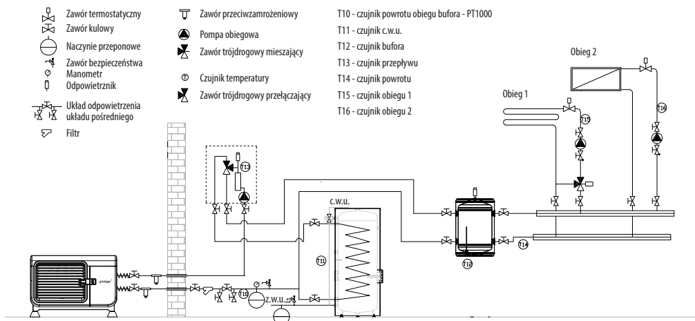
Rys. 66. Poglądowy schemat hydrauliczny instalacji z pompą ciepła Airmax 3 i modulem hydraulicznym Gbox
