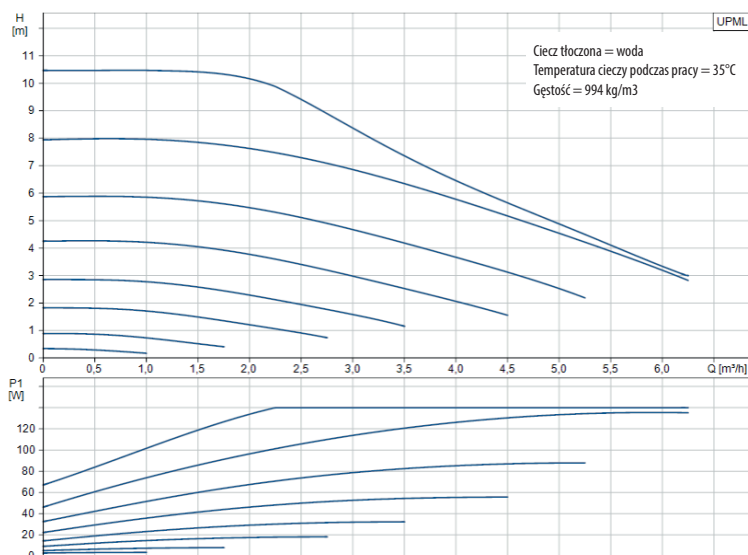
Wykres 8. Charakterystyki pompy obiegowej UPML GEO 25-105 130- czynnik: woda
