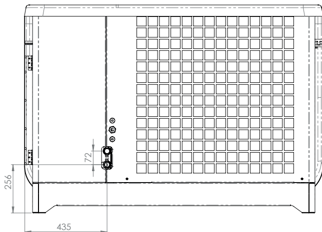
Rys. 13. Wymiary Airmax³ 7GT - widok z tyłu
