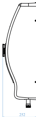
Rys. 21. Wymiary modułu Gbox - widok z boku
