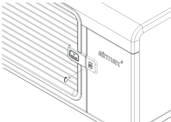
Rys. 55. Demontaż ściany przedniej Airmax³
