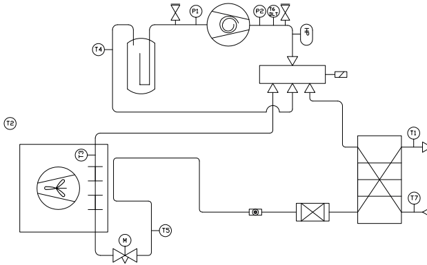
Rys. 14. Schemat chłodniczy pompy ciepła Airmax 3
