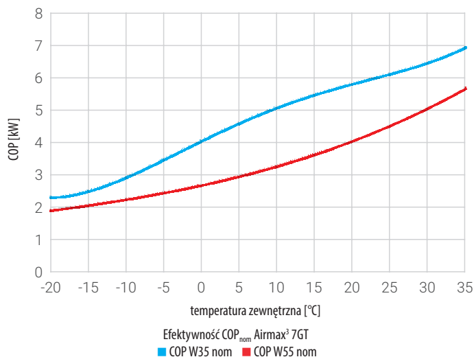
Wykres 4. COP (obroty nominalne sprężarki) dla zastosowań niskotemperaturowych (W35) i wysokotemperaturowych (W55) - pompa ciepła Airmax³ 7GT
